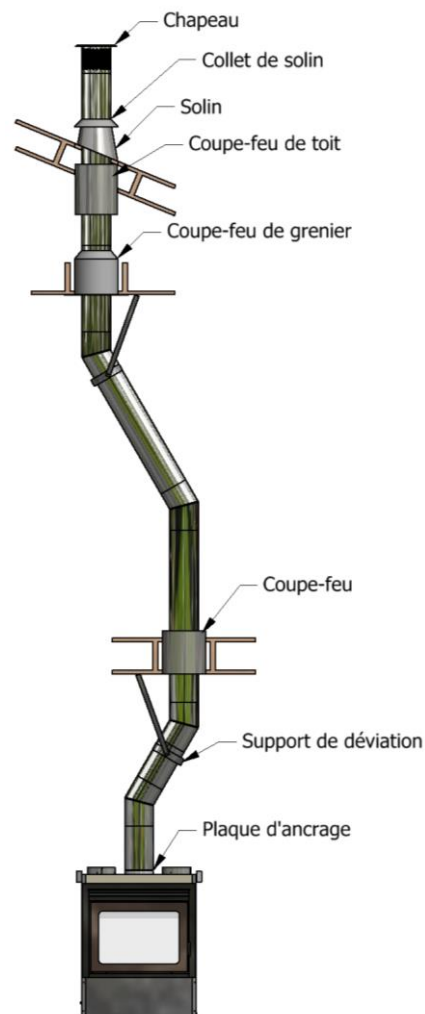
Illustration 18 – Installation de cheminée
