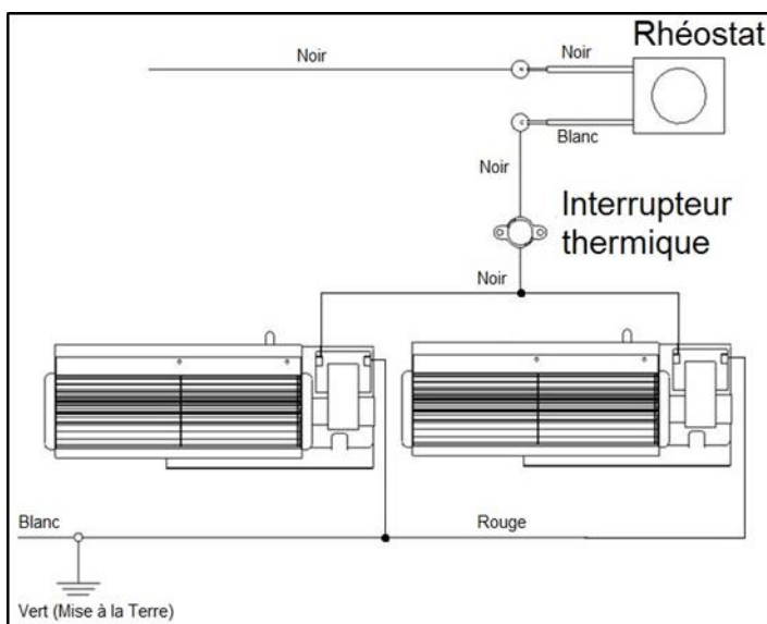
Illustration 17 – Branchements électriques du système de ventilation
