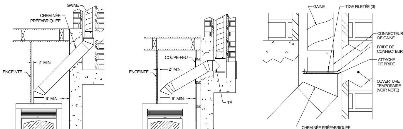
Illustration 20 – Connexion à une cheminée de maçonnerie
