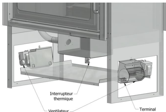
Illustration 16 – Emplacement du système de ventilation
