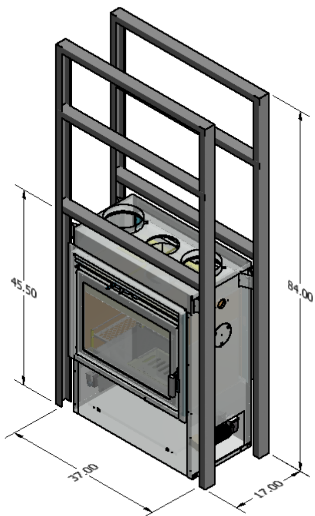
Illustration 11 – Dimensions minimales de l'ossature
